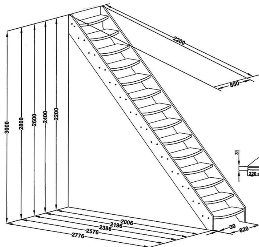
Схема Лестница прямая, 14 ступеней (15 подъемов по 200 мм)
