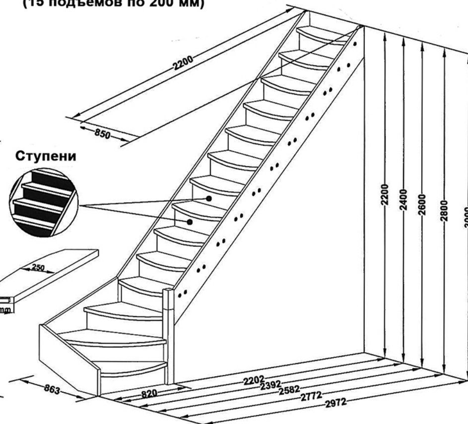
Схема Лестница с поворотом на 90°, 11 ступеней + 3 угловые ступени (15 подъемов по 200 мм)
